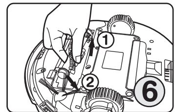
Pensez à nettoyer la structure du rouleau
