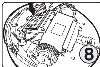
Placez convenablement le cadre
