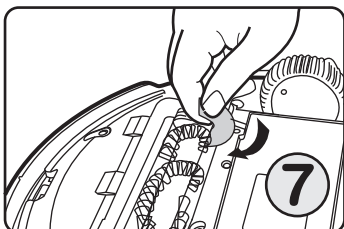
Remplacez la brosse dans le robot
